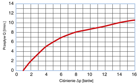
CHECK VALVE® Krzywa przepływu – screened BR660080024100; T = 50 °C, olej hydrauliczny HLP46
