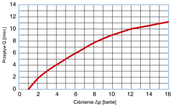
CHECK VALVE® Krzywa przepływu – unscreened BF660080024100; T = 50 °C, olej hydrauliczny HLP46
