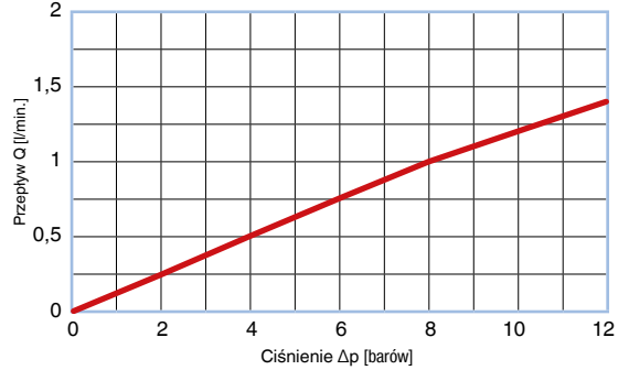
CHECK VALVE® Krzywa przepływu – screened BFAA055014; T = 50 °C, olej hydrauliczny HLP46
