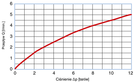
CHECK VALVE® Krzywa przepływu – unscreened BFAA055U014; T = 50 °C, olej hydrauliczny HLP46
