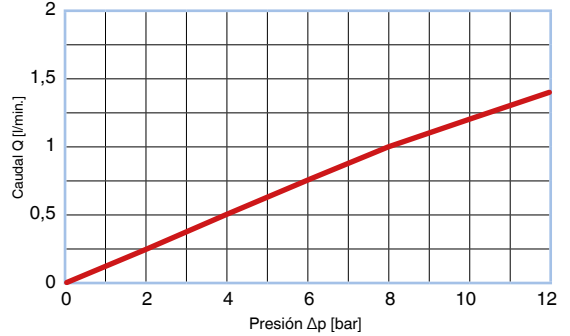
Curva caudal-presión, CHECK VALVE® – con tamiz BFAA055014; T = 50 °C, Aceite hidráulico HLP46
