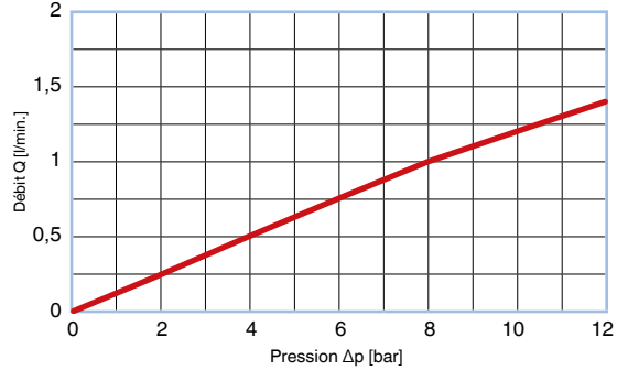
CHECK VALVE® Courbe de flux – screened BFAA055014; T = 50 °C, huile hydraulique HLP46
