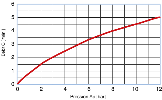
CHECK VALVE® Courbe de flux – unscreened BFAA055U014; T = 50 °C, huile hydraulique HLP46
