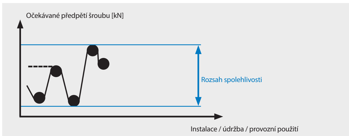
Obrázek 3 Očekávané předpětí
