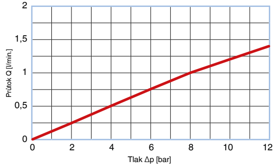
CHECK VALVE® Křivky průtoku – screened BFAA055014; T = 50 °C, hydraulický olej HLP46
