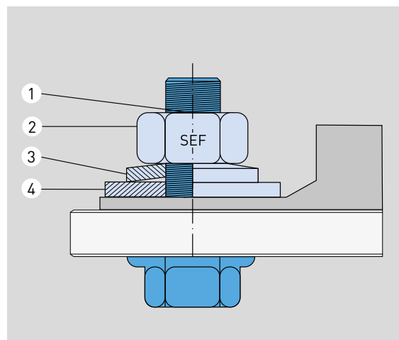
Quatre éléments fonctionnels en un = ecosyn®-SEF 1. Raccord fileté | 2. Écrou | 3. Disque de serrage | 4. Rondelle
