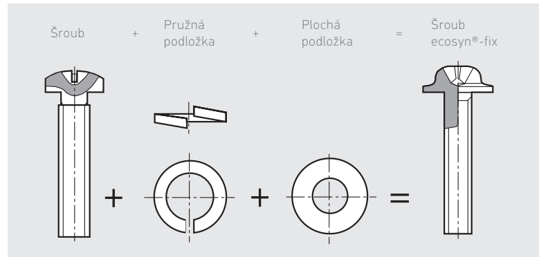
Jeden spojovací prvek namísto několika
