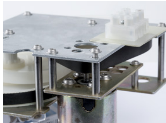
Příklad spoje za použití šroubů ecosyn®-fix na části čerpadla.
